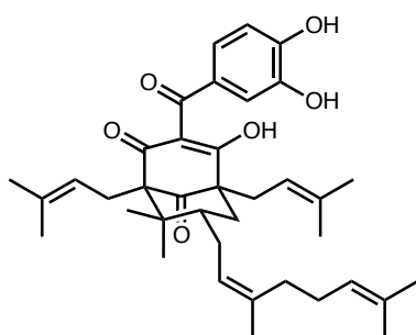
oblongifolin B (167)
