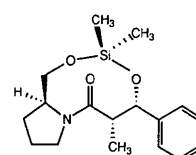
syn -Diastereomer (II)
